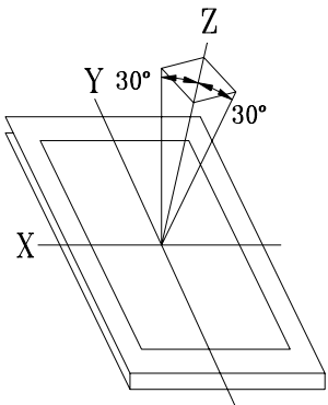
从Z轴距X, Y轴 \phi=30^\circ , 距离 30\pm 5\text{cm} 范围内检验。
